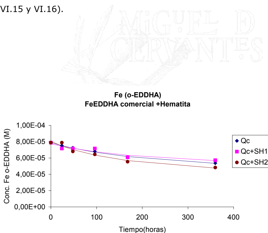
Fig.VI.21. Evolución de la concentración Fe quelado tras la interacción de Qc, Qc+SH1 y Qc+SH2 con hematita, con el paso del tiempo.
