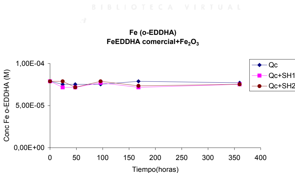
Fig.VI.16. Evolución de la concentración Fe (o-EDDHA) tras la interacción de Qc, Qc+SH1 y Qc+SH2 con óxido de Fe amorfo, con el paso del tiempo.
