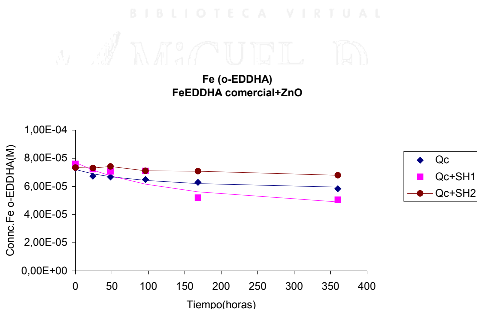
Fig.VI.38. Variación de la concentración de Fe (o-EDDHA) frente al tiempo para Qc, Qc+SH1 y Qc+SH2 que ha interactuado con óxido de Zn.
