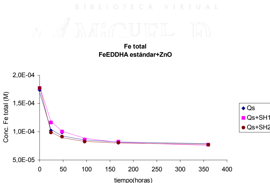
Fig.VI.36. Variación de la concentración de Fe total frente al tiempo para Qs, Qs+SH1 y Qs+SH2 que ha interactuado con óxido de Zn.
