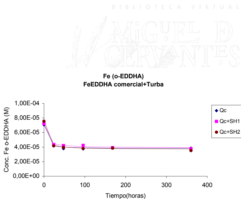
Fig.VI.57. Variación de la concentración de Fe (o-EDDHA) frente al tiempo para Qc, Qc+SH1 y Qc+SH2 que ha interactuado con Turba.
