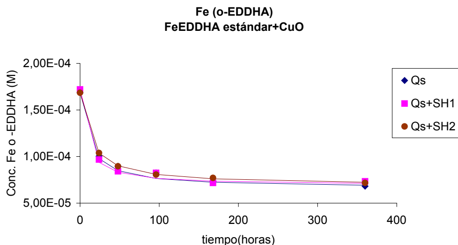
Fig.VI.24. Variación de la concentración de Fe (o-EDDHA) frente al tiempo para Qs, Qs+SH1 y Qs+SH2 que ha interactuado con óxido de Cu.
