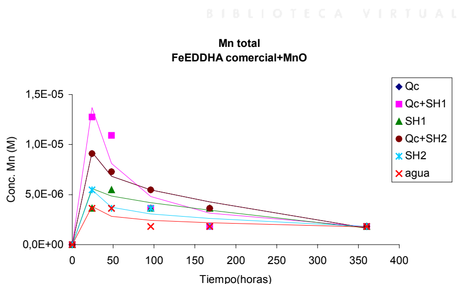
Fig.VI.50. Variación de la concentración de Mn frente al tiempo para Qc, Qc+SH1, Qc+SH2, SH1, SH2 y agua que ha interactuado con óxido de Mn.
