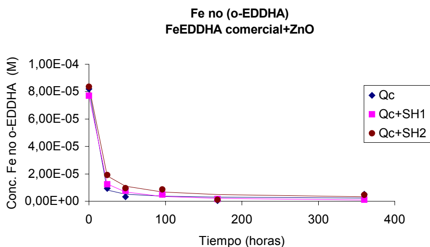
Fig.VI.40. Variación de la concentración de Fe no (o-EDDHA) frente al tiempo para Qc, Qc+SH1 y Qc+SH2 que ha interaccionado con óxido de Zn.
